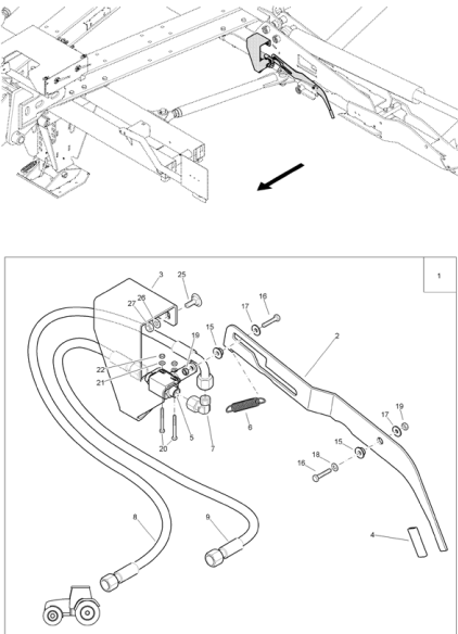
E0401 Hydraulikplan: Gebläse mit Kühler Seite 100
