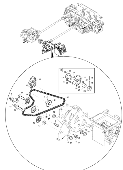
D0205 Kettenverlauf (5) Seite 88
