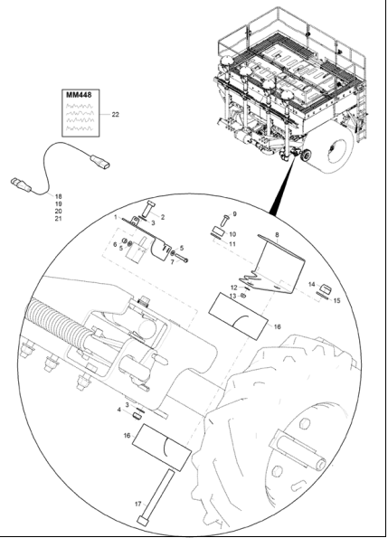
F0502 Saatleitungsüberwachung (2) Seite 142
