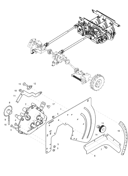
D0202 Kettenverlauf (2) Seite 82
