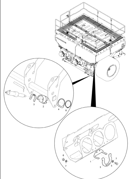
N0102 Exaktstriegel 15 mm DMC 12001-2C (2) bis 02.2018 Seite 242
