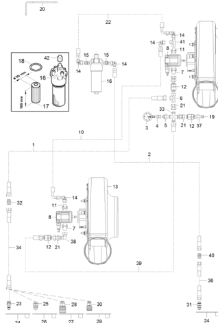
E0402 Hydraulikplan: Gebläse ohne Kühler Seite 102
