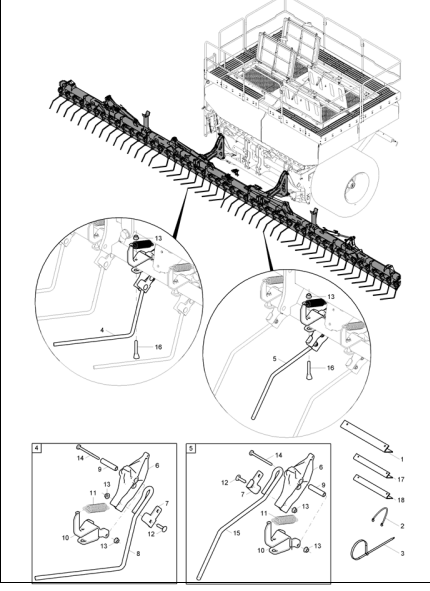
N0105 Exaktstriegel DMC 12M (1) ab 03.2018 Seite 248
