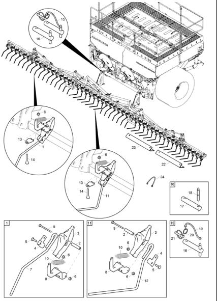
N0103 Exaktstriegel 15 mm DMC 12001-2C (3) bis 02.2018 Seite 244
