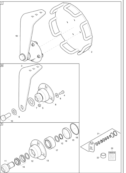
J0202 Bügelrolle Guss wartungsfrei Seite 216
