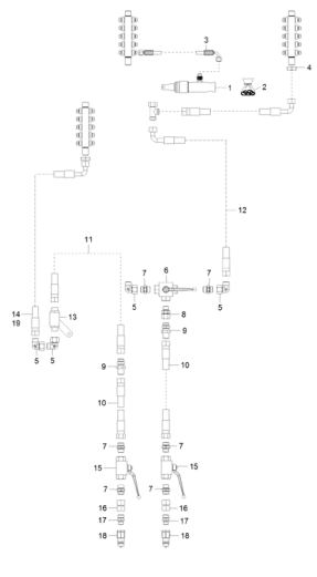
E0404 Hydraulikplan: Klappsperrung / Reibradhalterung / Deichsel Seite 106
