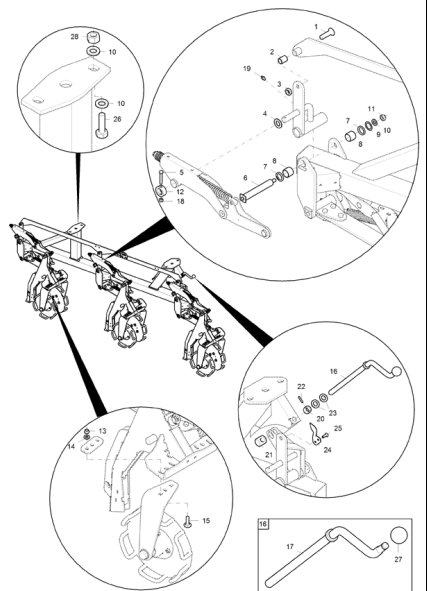
J0122 Scharhalter 3re. -1li. -250 (25 cm) (2) Seite 208
