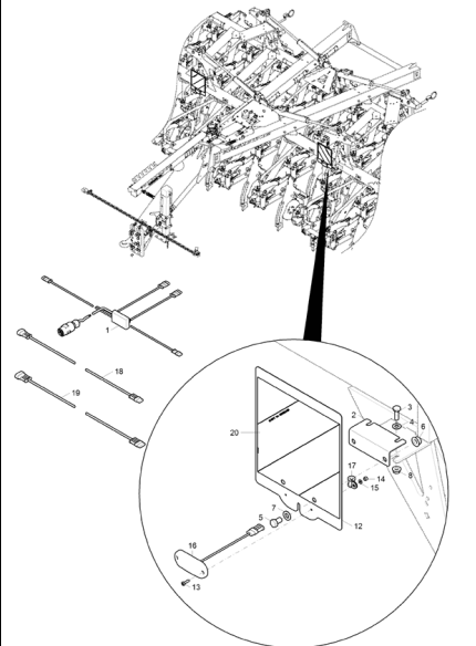
F0501 Saatleitungsüberwachung (1) Seite 140
