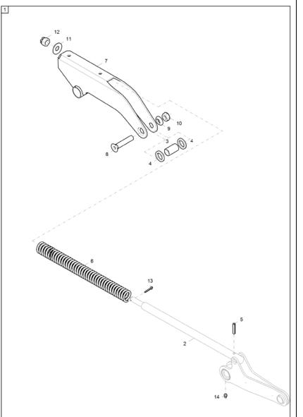
J0123 Scharhalter 3re. -1li. -250 (25 cm) (3) Seite 210
