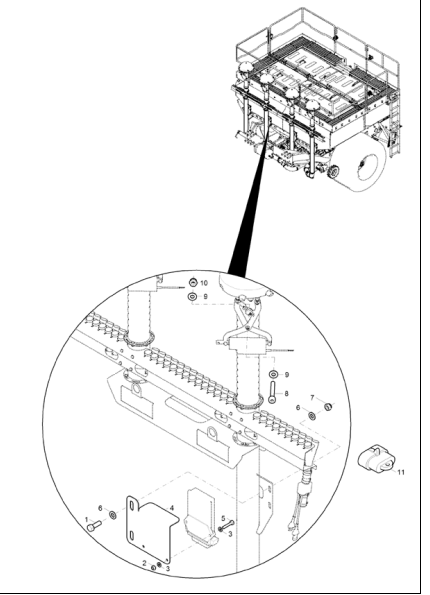
F0503 Saatleitungsüberwachung (3) Seite 144
