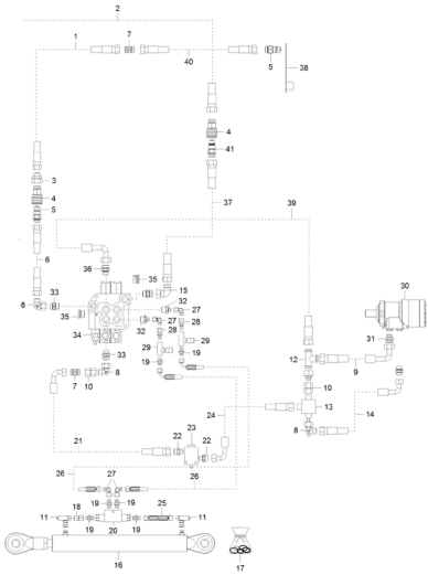
E0403 Hydraulikplan: Befüllschnecke Seite 104
