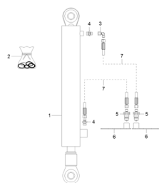
E0405 Hydraulikplan: Stellfuß DMC 12001-2C Seite 108
