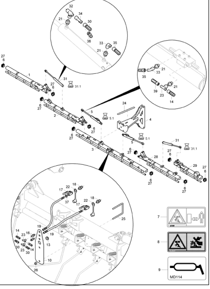
N0106 Exaktstriegel DMC 12M (2) ab 03.2018 Seite 250
