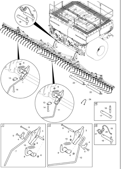
N0104 Exaktstriegel 15 mm DMC 12001-2C (4) bis 02.2018 Seite 246
