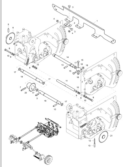
D0203 Kettenverlauf (3) Seite 84
