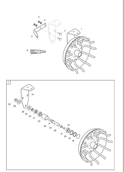
J0201 Steinbodenrolle Seite 214
