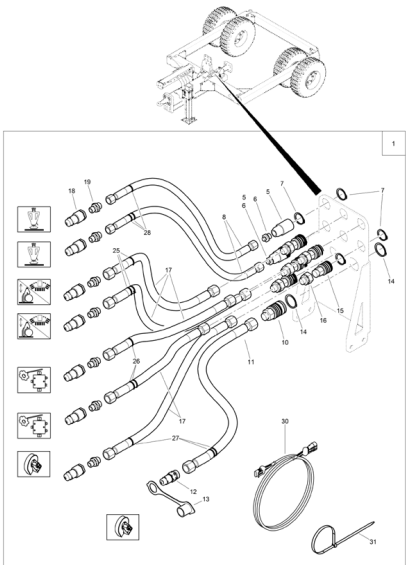
E0104 Reduzierstücke Seite 98
