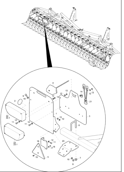
F030401 LED Arbeitsbeleuchtung Seite 138
