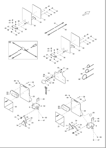
F030303 Verlängerungs-Set Beleuchtung Seite 136
