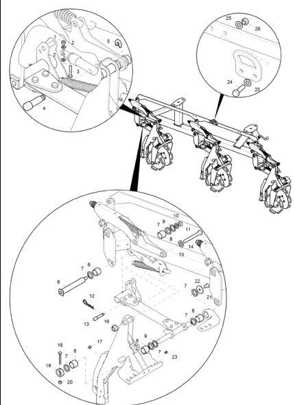
J0121 Scharhalter 3re. -1li. -250 (25 cm) (1) Seite 206
