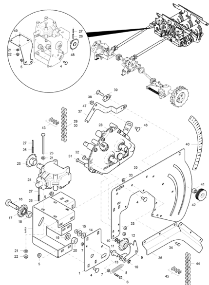
D0201 Kettenverlauf (1) Seite 80
