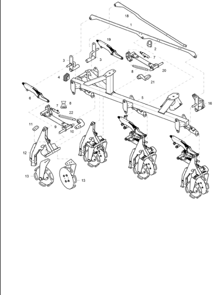
J0124 Scharhalter 3re. -1li. -250 (25 cm) (4) Seite 212
